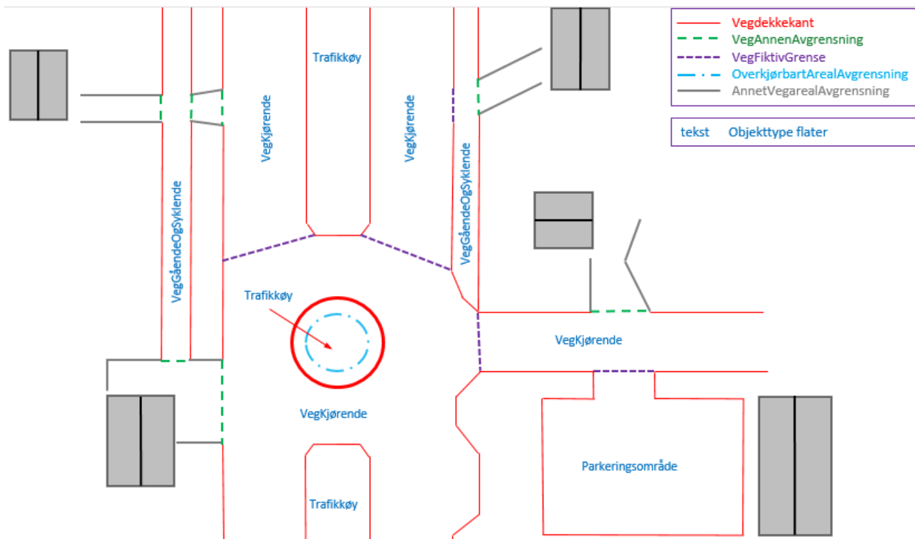
Figur 2. Eksempel på flater og avgrensningslinjer
