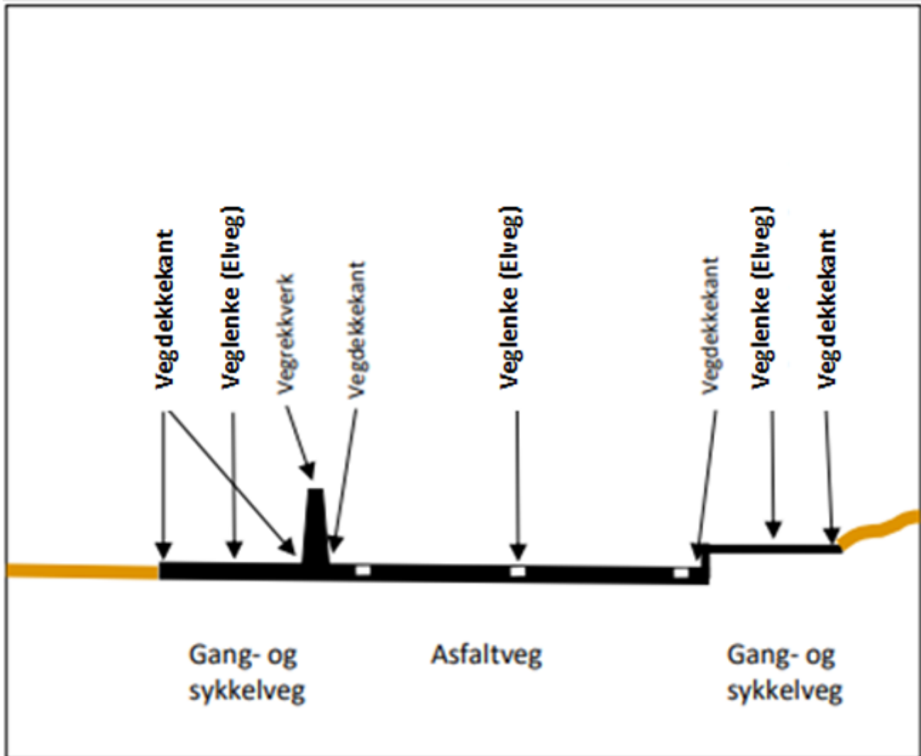
Figur 14. Eksempel på registrering av Gang- og Sykkelveg langs veg.
