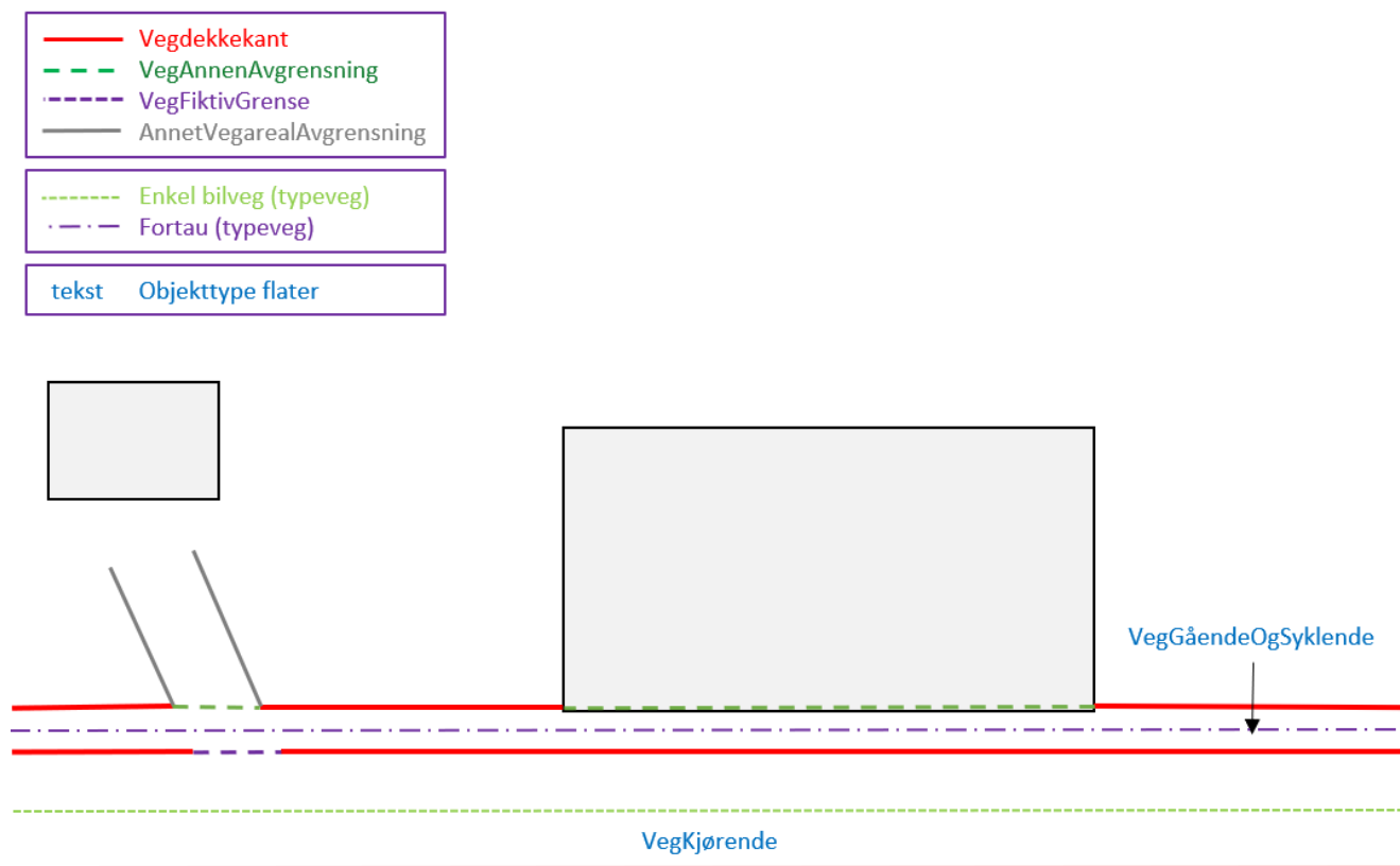
Figur 11. Eksempel på registrering av fortau som går mot bygning/husvegg. Egenskap Typeveg tilhører Elveg.
