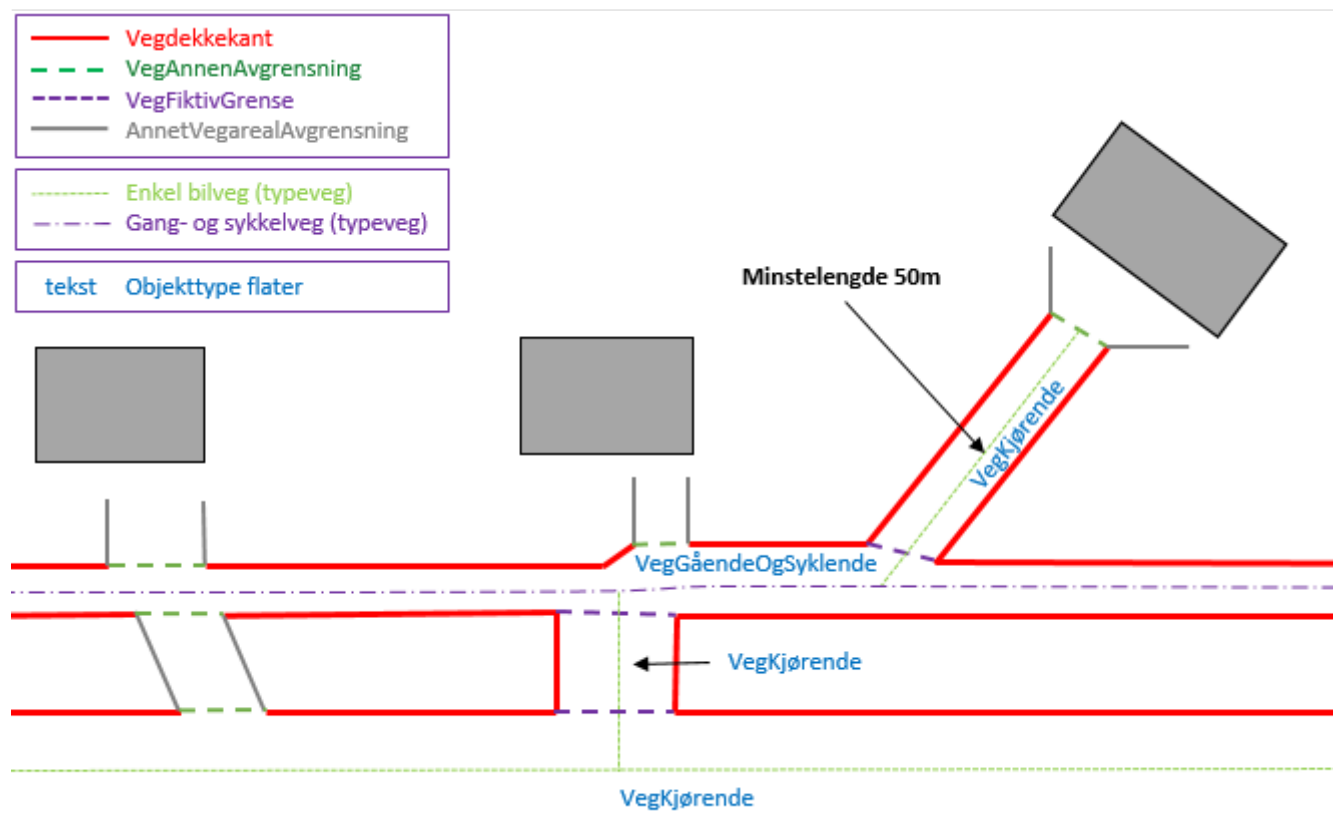
Figur 13. Eksempel på registrering av gang- og sykkelveg. Egenskap Typeveg tilhører Elveg.
