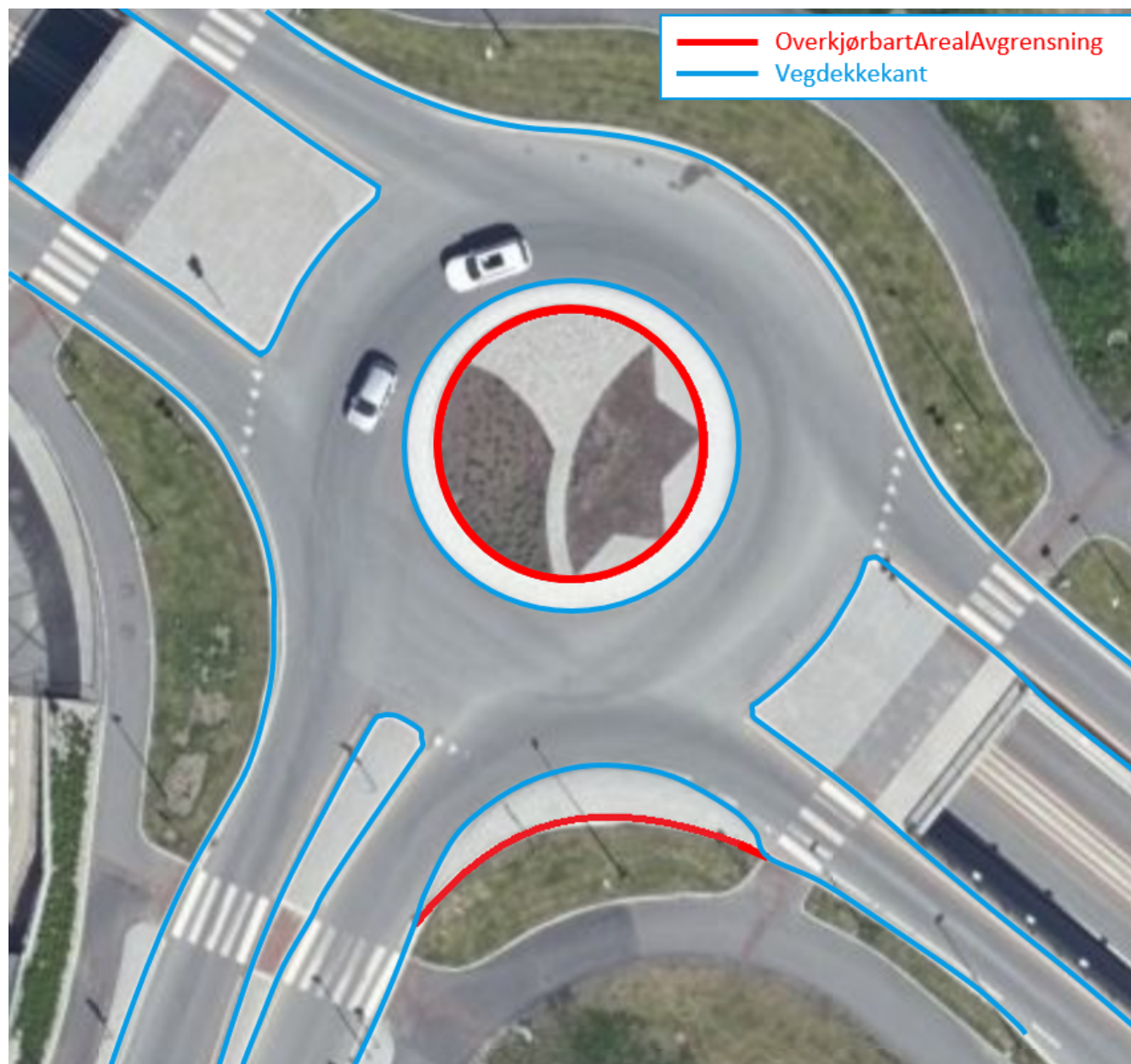
Figur 55. Illustrasjon fra produktspesifikasjon av OverkjørbartArealAvgrensning
