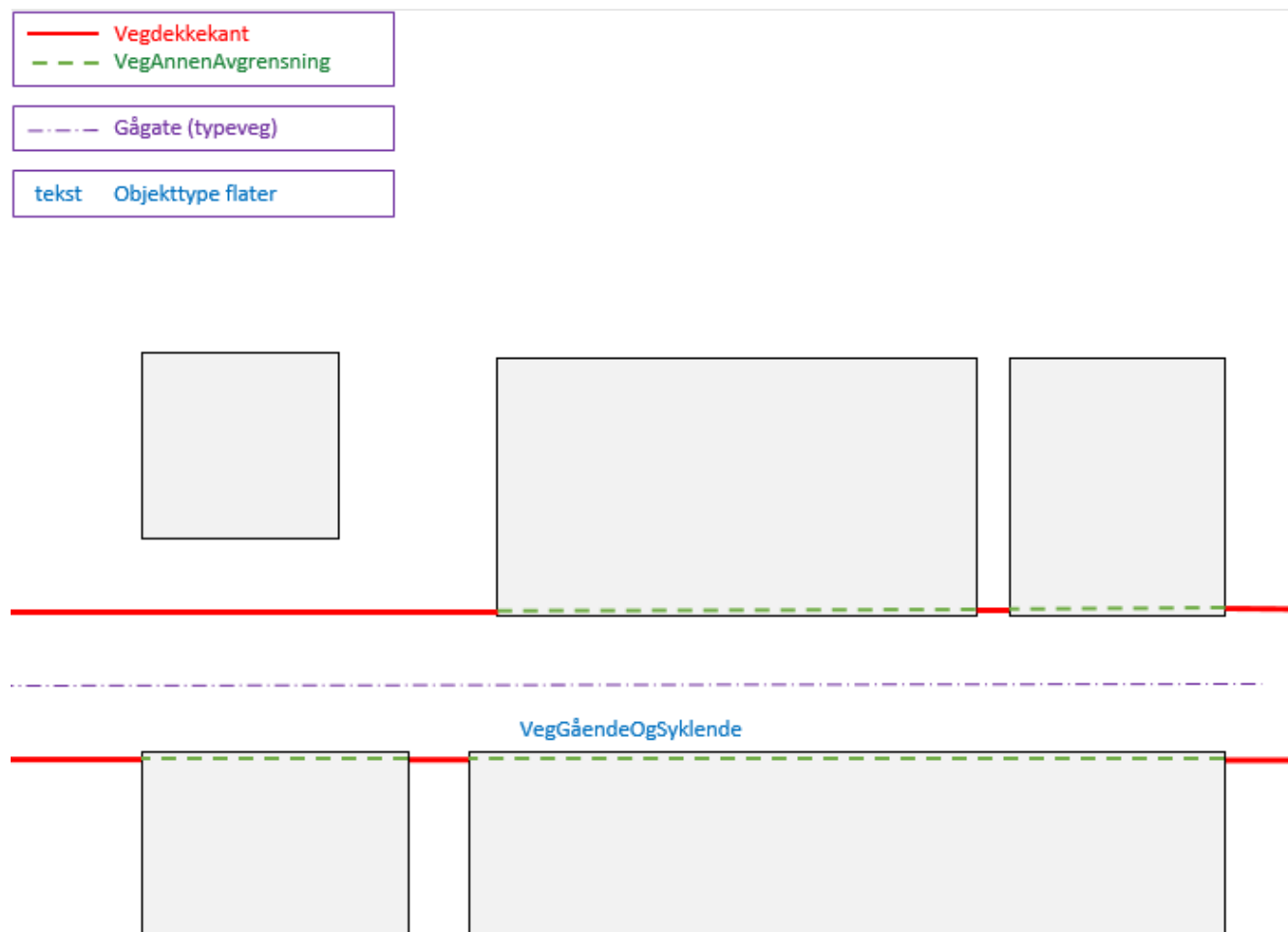
Figur 12. Eksempel på registrering av gågate som går mot bygning/husvegg. Egenskap Typeveg tilhører Elveg.
