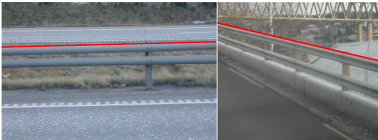
Figur 62. Illustrasjon fra produktspesifikasjon av Vegrekkverk
