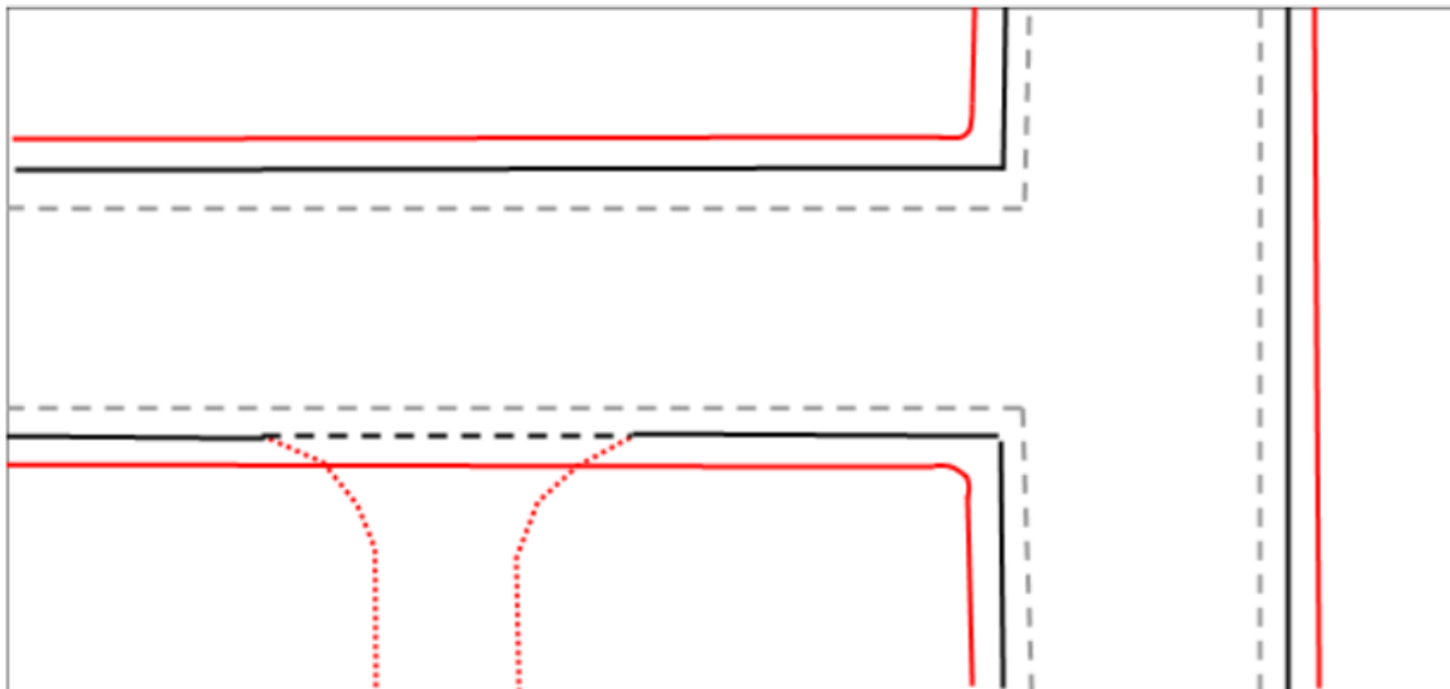
Figur 68. Eksempel på registrering av objekttype Vegskulderkant ved avkjørsel og vegkryss. I dette tilfellet har Kjørebane kant, Vegdekke kant og Vegskulderkant ulik geometri. Vegskulderkant er tegnet med rød heltrukken strek og skal registreres gjennomgående. Kjørebane kant er tegnet i grå stiplet farge, Vegdekke kant er tegnet med svart heltrukken strek, VegAnnenAvgrensning er tegnet med svart stiplet linje og AnnetVegarealAvgrensning er tegnet med rød prikket linje.
