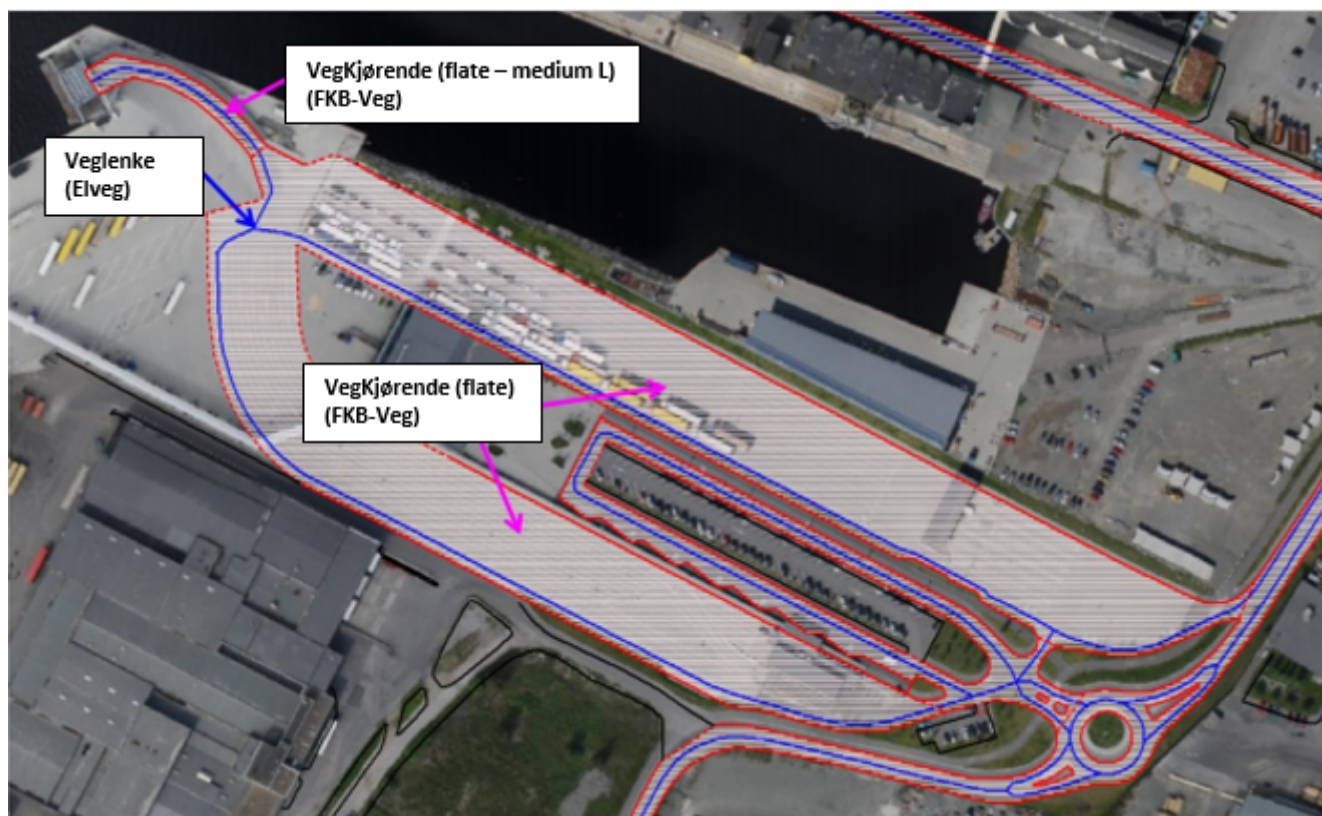
Figur 23. Eksempel på registrering av VegKjørende i forbindelse med fergeleie. Veglenke fra Elveg er her korrekt benyttet som manus for avgrensning av vegflatene.
