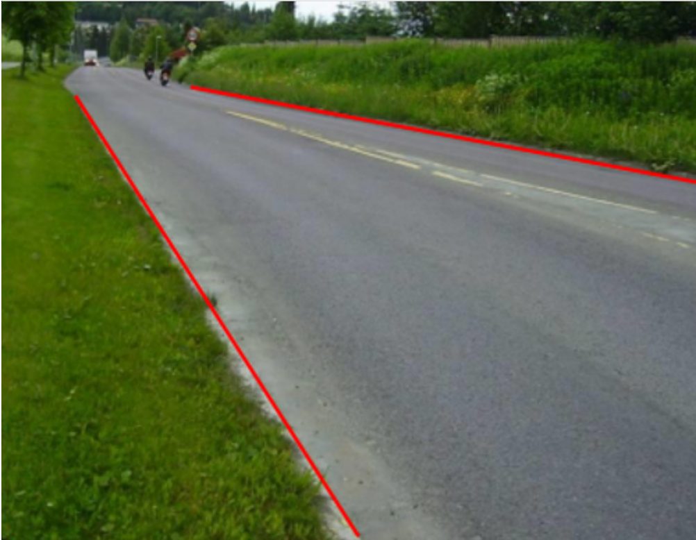
Figur 37. Eksempel på registrering av Vegdekkekanthorizont (rød strek). I dette tilfellet vil Vegskulderkant, Vegdekkekanthorizont og Kjørebanehorizont ha lik geometri i grunnriss og høyde (dersom opsjoner er bestilt).
