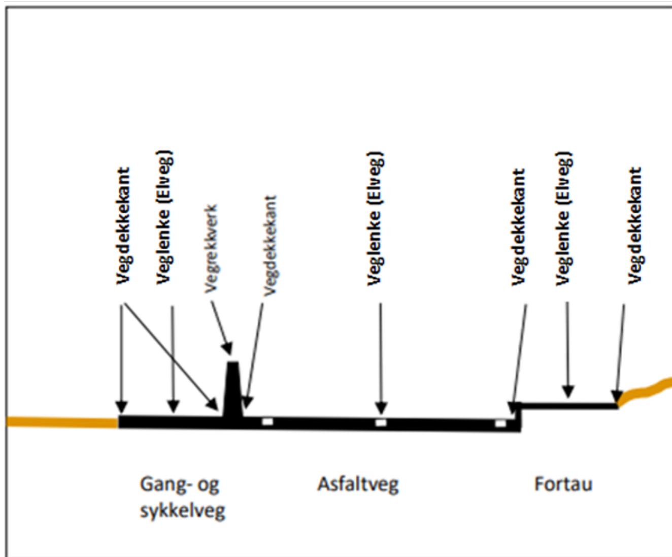
Figur 15. Eksempel på registrering av Gang- og Sykkelveg og Fortau langs veg.
