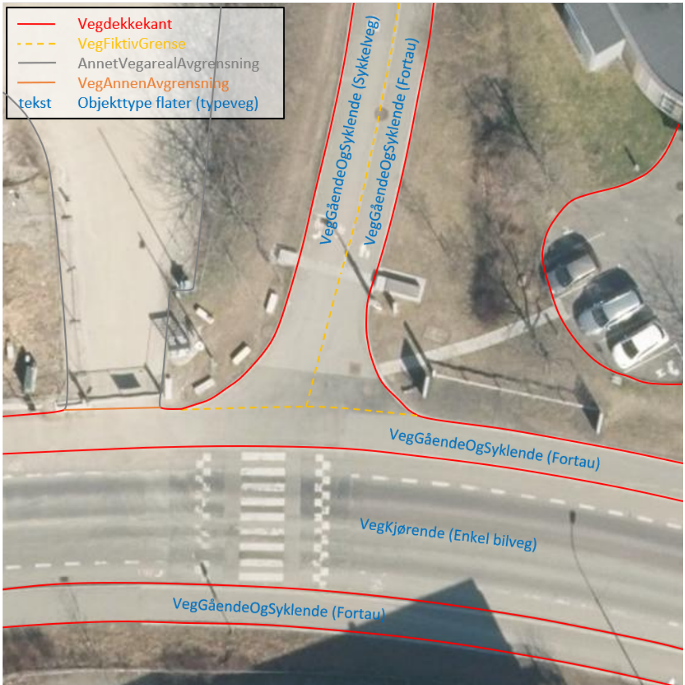
Figur 16. Eksempel på registrering av sykkelveg og gangveg uten fysisk skille mellom seg (kun oppmerking).
