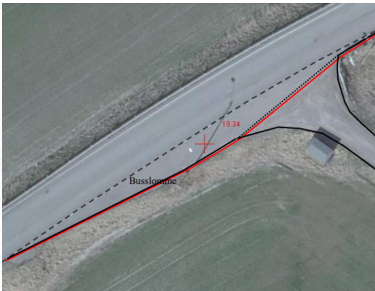
Figur 65. Eksempel på registrering av busslomme ved vegkryss. Grå stippet strek er Kjørebane kant. Svart strek er Vegdekkekant. Rød strek er Vegskulderkant. Svart prikket strek er VegAnnenAvgrensning.
