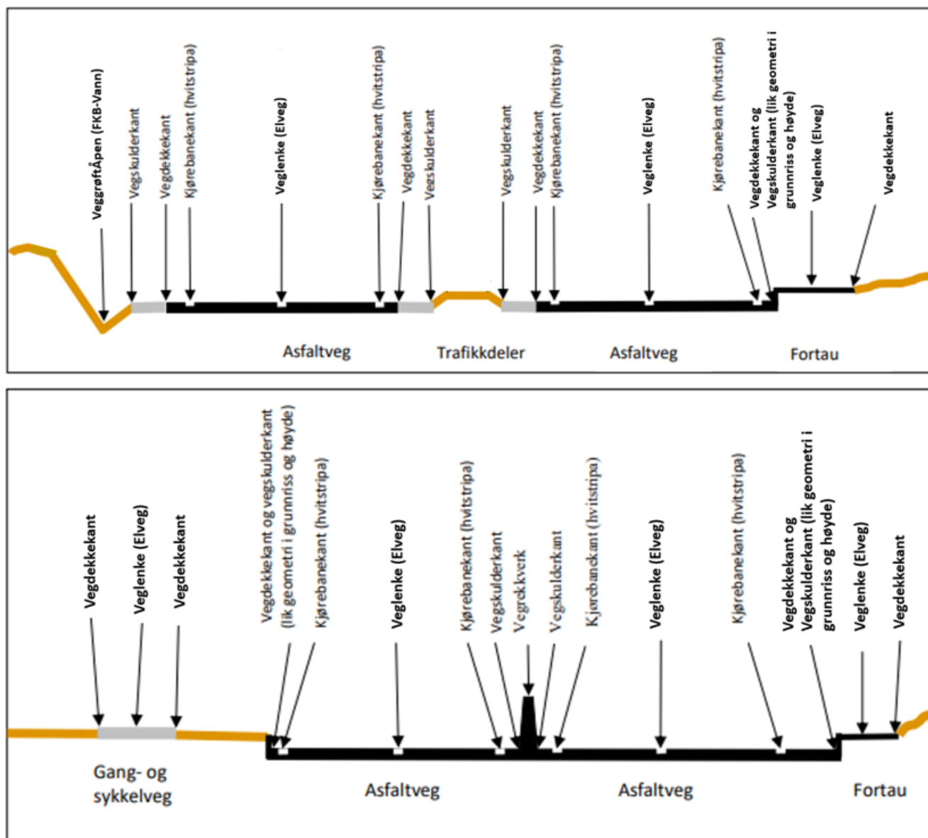
Figur 1. Eksempel på registrering av veg i SOSI/FKB versjon 5.0
