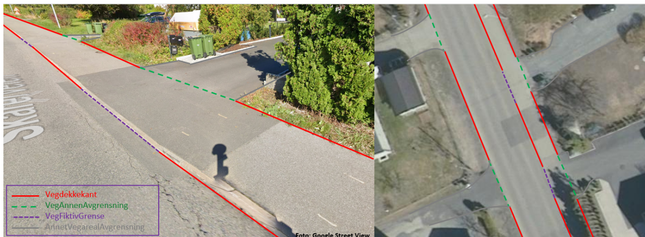
Figur 43. Eksempel på riktig registrering av VegFiktivGrense og VegAnnenAvgrensning i forbindelse med avkjørsel over fortau.
