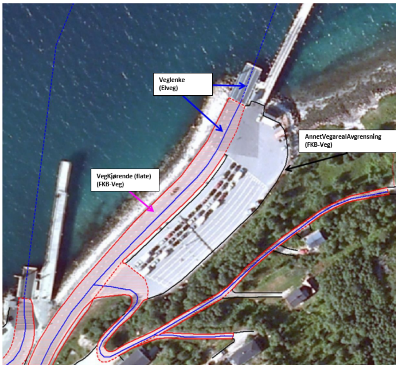
Figur 24. Eksempel på registrering av VegKjørende i forbindelse med et mindre fergeleie. Veglenke fra Elveg er her korrekt benyttet som manus for avgrensning av vegflatene.
