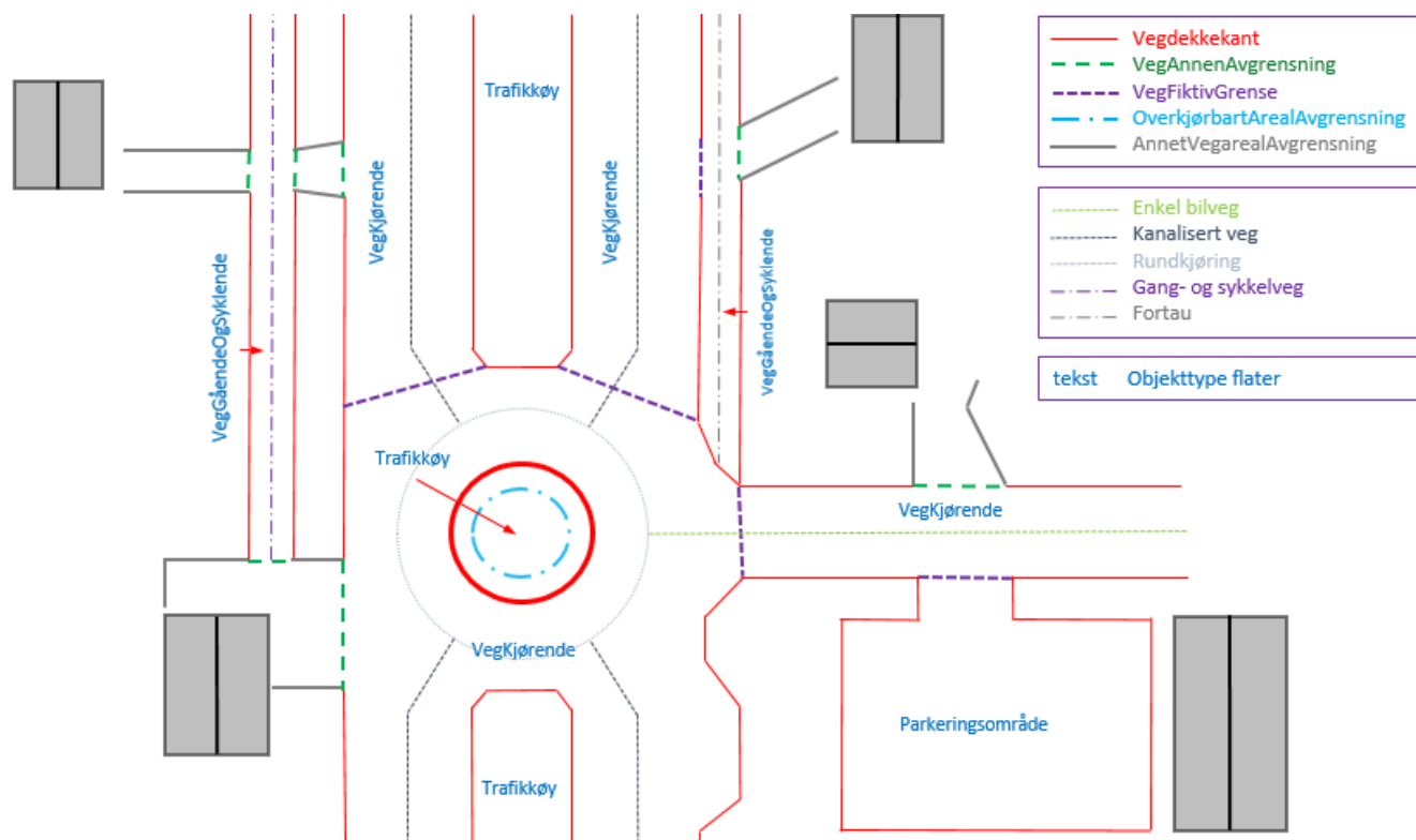
Figur 3. Eksempel på forholdet mellom flater og avgrensningslinjer i FKB-Veg og veglenker i Elveg 2.0
